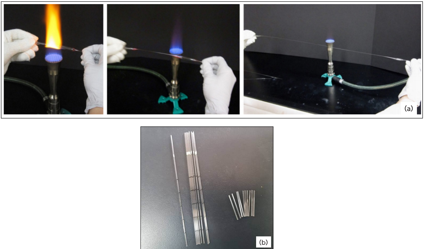
รูปที่ 3-7 (a) แสดงการทำหลอด capillary ใช้เอง (ที่มา: Nichols, 2025) และ (b) หลอด capillary สำเร็จรูปแบบมีสเกลและไม่มีสเกล
