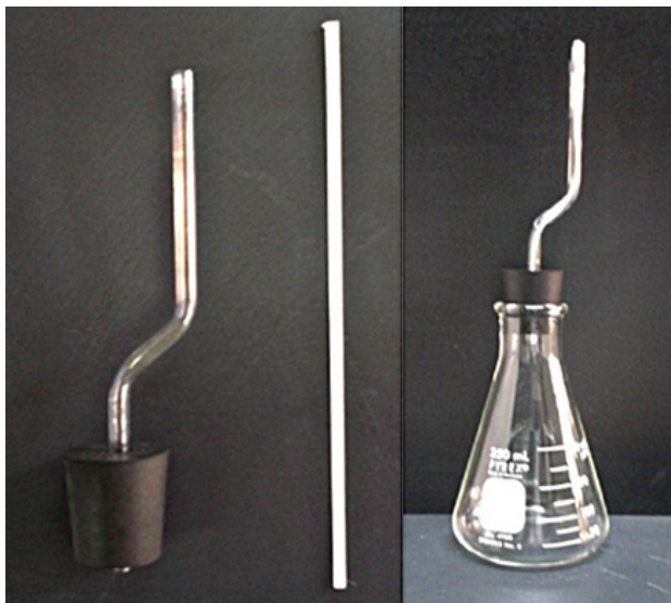
รูปที่ 10-4 อุปกรณ์สำหรับใช้ตรวจวิเคราะห์ไซยาไนด์ โดยวิธี Paper Strip Test
