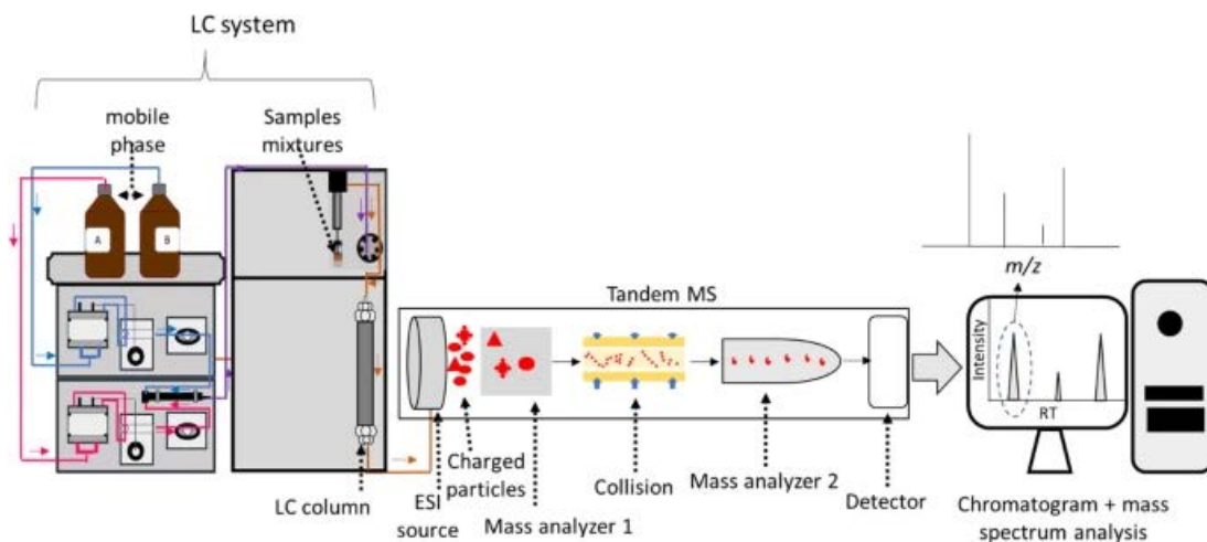
รูปที่ 3-13 Liquid chromatography–tandem mass spectrometry (LC–MS/MS) principles
