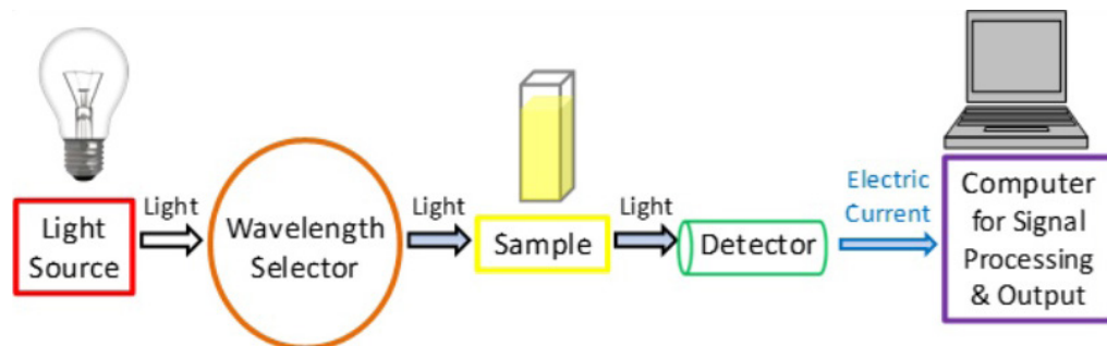
รูปที่ 3-10 ส่วนประกอบของเครื่อง UV-Vis spectrophotometer
