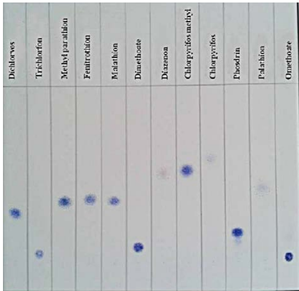
รูปที่ 4-8 TLC Chromatogram ของสารมาตรฐานกลุ่ม Organophosphates (OPs)
