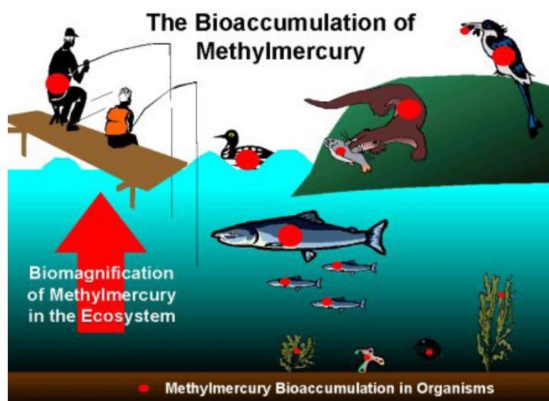
รูปที่ 9-2 Biomagnification ของ Methyl mercury ในระบบนิเวศน์ ที่มา: https://joshgitalis.com/wp-content/uploads/2012/08/i-f-bom-e.jpg
