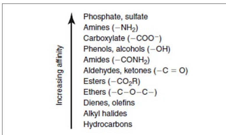
รูปที่ 3-2 แสดงการเกิดสัมพรรคภาพของ functional group ต่าง ๆ กับเฟสอยู่กับที่ชนิด silica gel ที่มา: Cai (2014)
