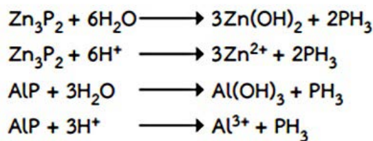
รูปที่ 6-2 การเกิดแก๊สฟอสฟีน ( \text{PH}_3 ) จากซิงค์ฟอสไฟด์ ( \text{Zn}_3\text{P}_2 ) และอะลูมิเนียมฟอสไฟด์ (ALP) หลังทำปฏิกิริยากับน้ำหรือกรด ที่มา: Proudfoot et al. (2009)
