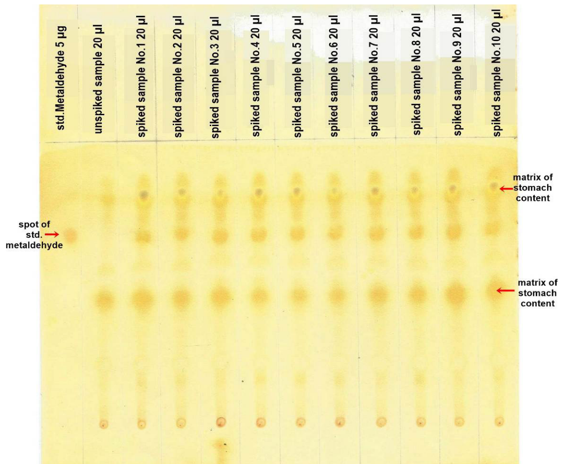
รูปที่ 7-4 TLC Chromatogram ของการทดสอบหาค่า LOD ของวิธีตรวจหา metaldehyde ในอาหารในกระเพาะ
