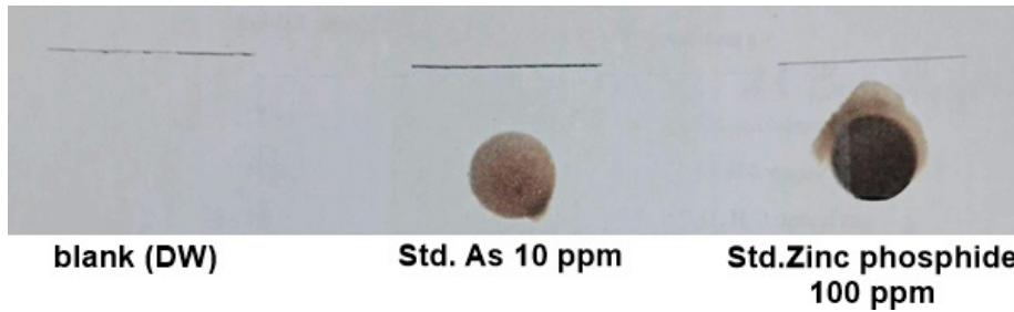
รูปที่ 9-3 แสดงผลบวกของสารมาตรฐาน As และ Zinc phosphide จากการตรวจวิเคราะห์หาสารกำจัดหนู โดย Gutzeit test
