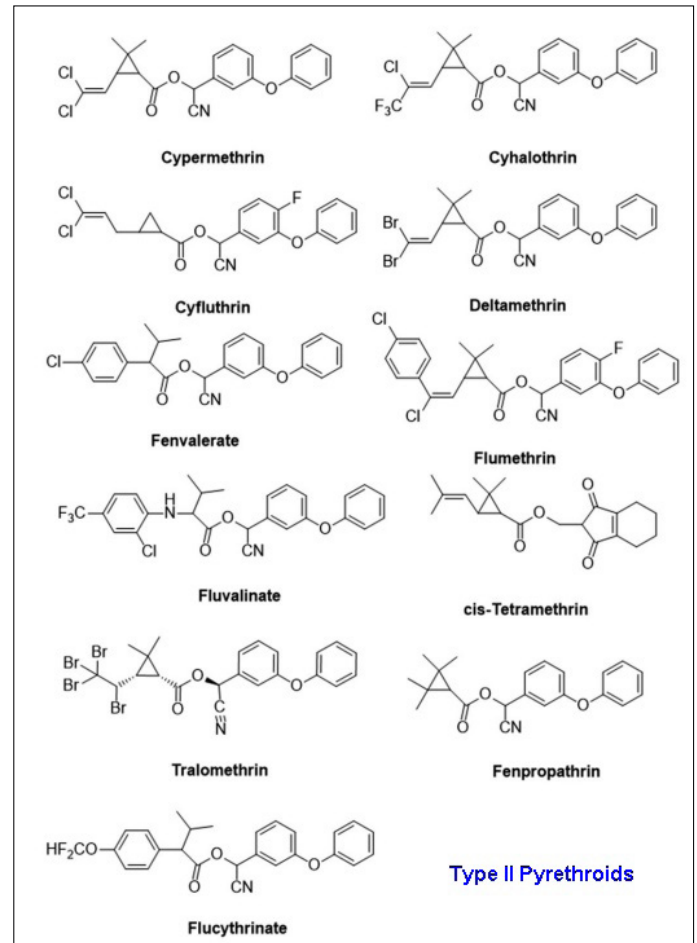
รูปที่ 4-7 ตัวอย่างสูตรโครงสร้างของ Type I Pyrethroids และ Type II Pyrethroids ที่มา: Ravula and Yenugu (2021)
