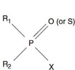
รูปที่ 4-1 สูตรโครงสร้างทั่วไปของสารเคมีกำจัดแมลงกลุ่ม Organophosphates ที่มา: Klaassen (2013)
