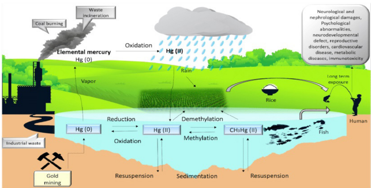
รูปที่ 9-1 Mercury Cycle ที่มา: Busairi & Syahir (2018)
