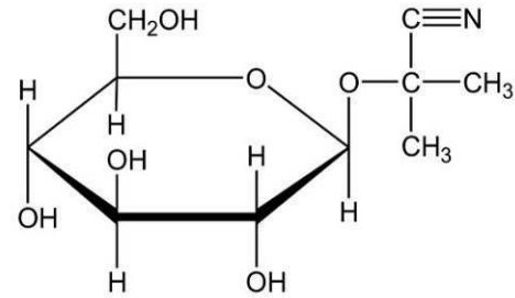
รูปที่ 10-2 สูตรโครงสร้างของ linamarin
