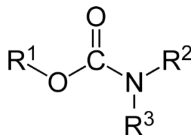
รูปที่ 4-3 สูตรโครงสร้างทั่วไปของสารเคมีกำจัดแมลงกลุ่ม Carbamates ที่มา: https://commons.wikimedia.org/wiki/File:Carbamate-group-2D.png
