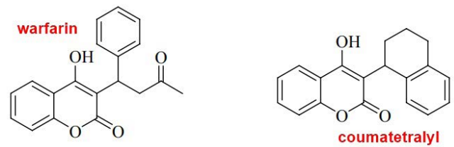
รูปที่ 6-5 สูตรโครงสร้างของ Warfarin และ Coumatetralyl
