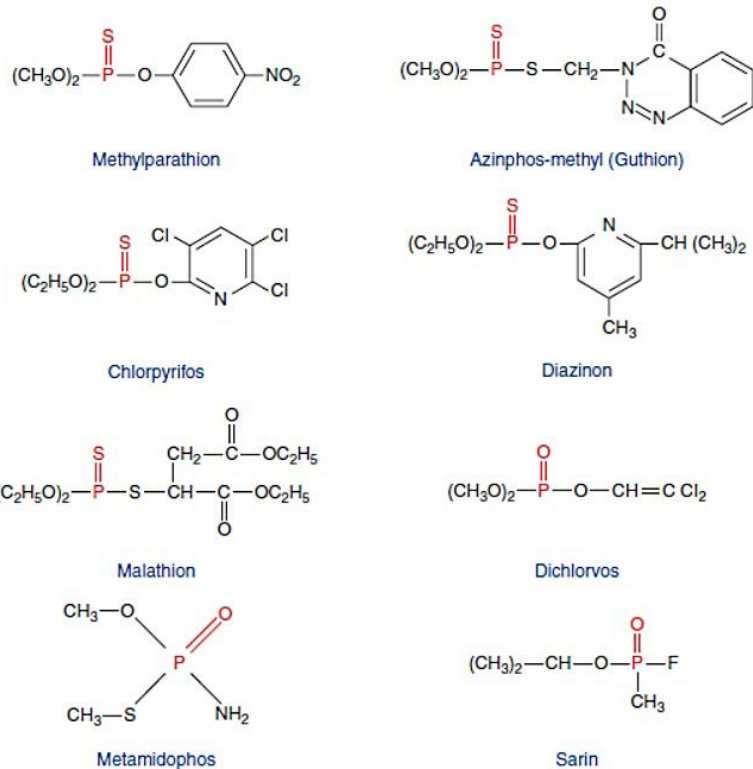
รูปที่ 4-2 ตัวอย่างสารเคมีกำจัดแมลงกลุ่ม Organophosphates บางชนิดและสารทำลายประสาทซาริน ที่มา: Klaassen (2013)
