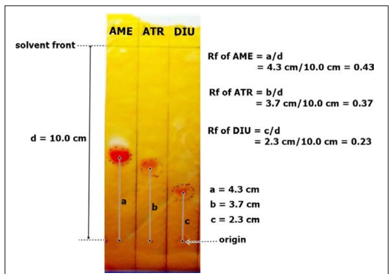
รูปที่ 3-9 ตัวอย่างการคำนวณหาค่า R_f ของสารละลายมาตรฐานกำจัดวัชพืชชนิด ametryn (AME), atrazine (ATR) และ diuron (DIU) บนแผ่น TLC
