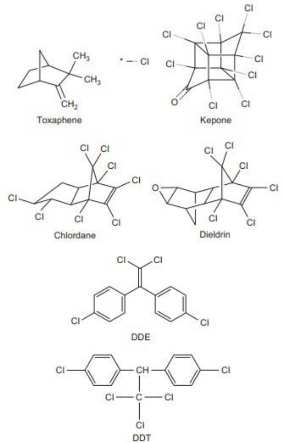
รูปที่ 4-6 ตัวอย่างสารเคมีกำจัดแมลงกลุ่ม Organochlorines ชนิดต่าง ๆ พร้อมสูตรโครงสร้าง ที่มา: Gupta (2018)
