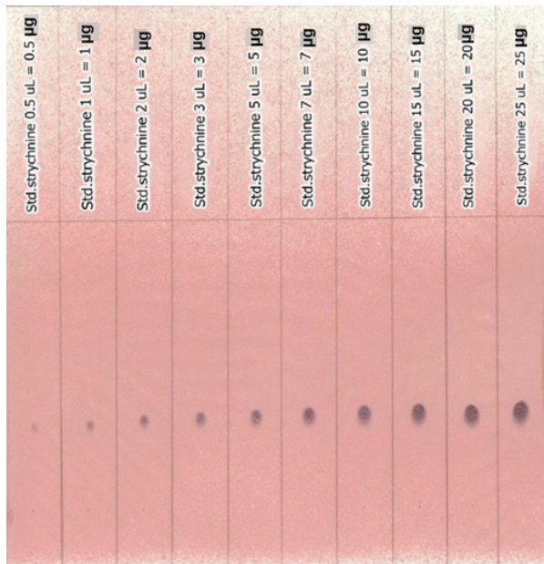
รูปที่ 6-4 TLC chromatogram ของสารละลายมาตรฐาน strychnine ที่ปริมาณต่าง ๆ กัน
