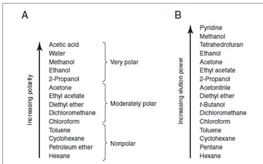
รูปที่ 3-3 A คือ ตัวทำละลายที่ใช้เป็น mobile phase ซึ่งพบได้บ่อย จัดเรียงตามลำดับความมีขั้วที่เพิ่มขึ้น
