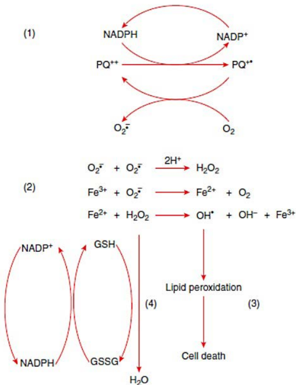
รูปที่ 5-2 กลไกการออกฤทธิ์ของพาราควอต
