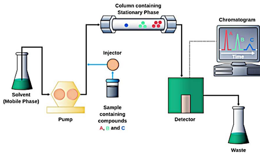
รูปที่ 3-11 Flow diagram ของการแยกสารด้วยเทคนิค HPLC ที่มา: https://theory.labster.com/niche_hplc/
