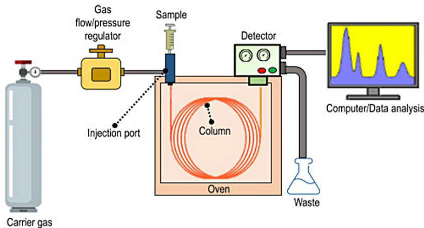
รูปที่ 3-12 ส่วนประกอบสำคัญของเครื่อง GC
