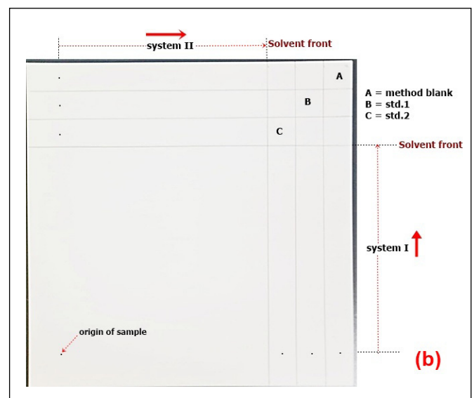
รูปที่ 3-6 การเตรียม TLC plate เพื่อตรวจวิเคราะห์สารพิษ (a) One-dimensional TLC (b) Two-dimensional TLC
