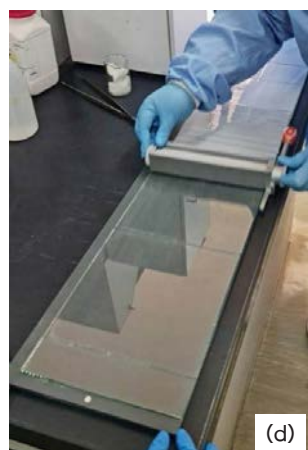
รูปที่ 3-5 วิธีการ coat plate (a) Silica gel 60 GF 254 และน้ำกลั่น (b) เช็ดกระจกด้วย acetone (c) เท Silica gel 60 GF 254 ที่ผสมด้วยน้ำกลั่นลงใน Moveable spreader (d) ค่อยๆลาก Moveable spreader ไปข้างหน้าสุดทาง และ (e) TLC ที่อบเรียบร้อยแล้ว เก็บในตู้เก็บ TLC plate
