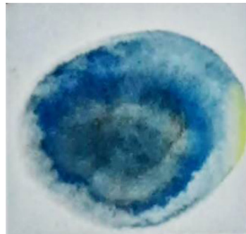
รูปที่ 9-4 สีน้ำเงินบนกระดาษกรอง จากการทำ Molybdenum blue test
