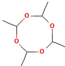
รูปที่ 7-1 สูตรโครงสร้างทางเคมีของ metaldehyde
