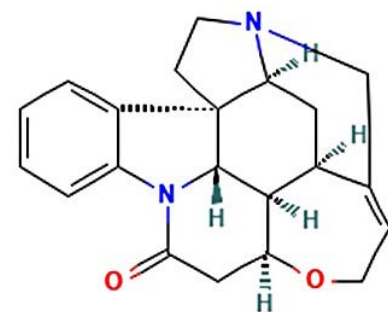
รูปที่ 6-3 สูตรโครงสร้างสตริกนิน
