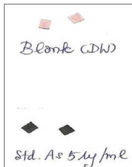
รูปที่ 9-5 ผลบวกของสารมาตรฐาน As จากการตรวจวิเคราะห์โดย Reinsch test
