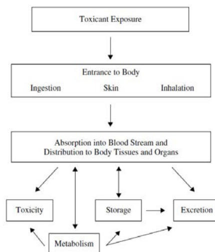
รูปที่ 1-6 กระบวนการเปลี่ยนแปลงต่าง ๆ ของสารพิษเมื่อเข้าสู่ร่างกาย (Toxicokinetics)
