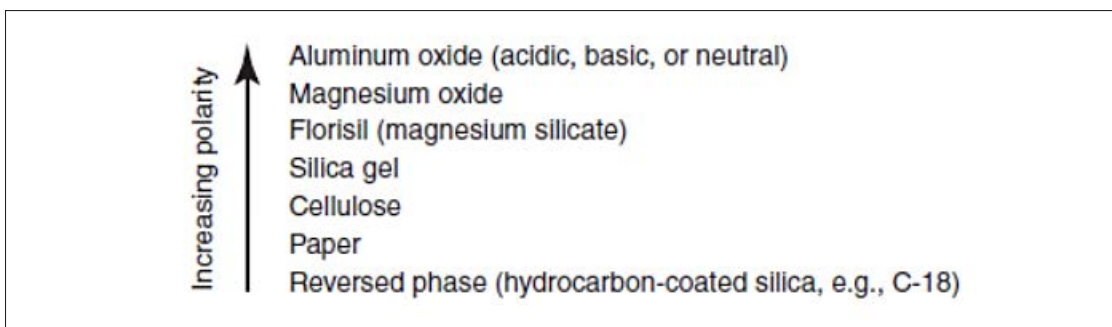
รูปที่ 3-1 แสดงความมีขั้วชนิดของเฟสอยู่กับที่ชนิดต่าง ๆ ของ TLC ที่มา: Cai (2014)
