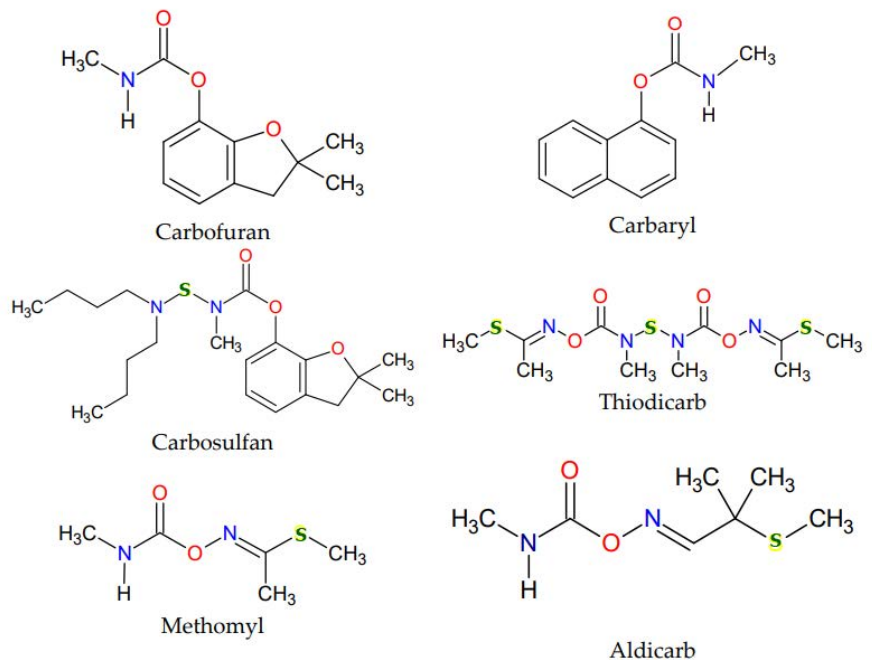
รูปที่ 4-4 สูตรโครงสร้างของสารเคมีกำจัดแมลงกลุ่ม Carbamates บางชนิด ที่มา: Pereira et al. (2023)
