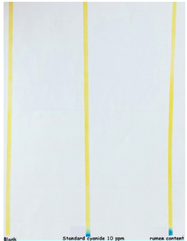
รูปที่ 10-5 การตรวจหาไซยาไนด์ในตัวอย่างอาหารในกระเพาะรูเมนด้วย วิธี paper strip test
