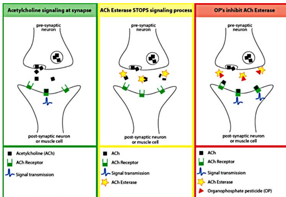
รูปที่ 4-5 กลไกการออกฤทธิ์ของสารเคมีกำจัดแมลงกลุ่ม Organophosphates โดยการยับยั้งการทำงานของเอนไซม์ acetyl cholinesterase (AChE)
