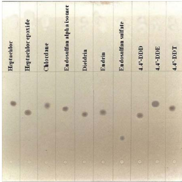
รูปที่ 4-10 TLC Chromatogram ของสารมาตรฐานกลุ่ม Organochlorines (OCs)
