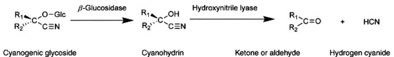
รูปที่ 10-3 การเปลี่ยนแปลงของไซยาโนเจนิกไกลโคไซด์จนเกิดไฮโดรเจนไซยาไนด์
