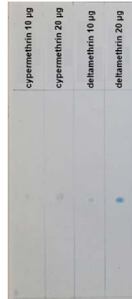
รูปที่ 4-11 TLC Chromatogram ของสารมาตรฐานกลุ่ม Pyrethroids (PYRs)
